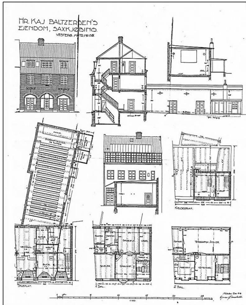
Arkitekt Ejnar Ørnsholts forslag til biografbygning, 1916
